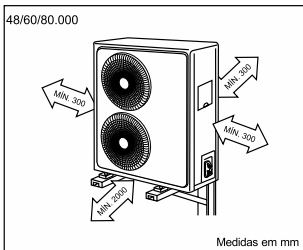
DISTÂNCIAS PARA FIXAÇÃO DA BASE DA UNIDADE CONDENSADORA
